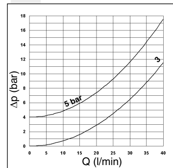
Curva n° 3 = Flusso pilotato
